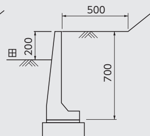
基礎工および 標準敷設図
