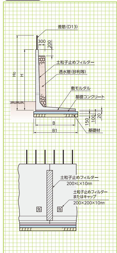
標準敷設図
