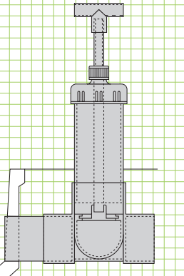
施工図 一般水路用
