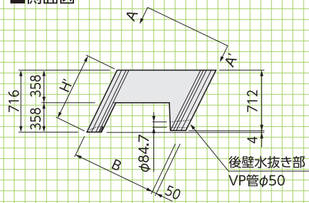
■側面図
