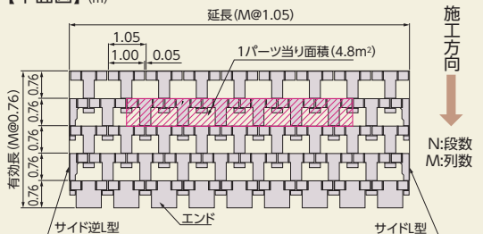
【平面図】(m)
