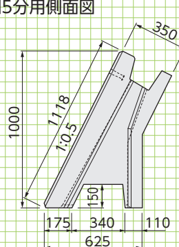
■5分用側面図
