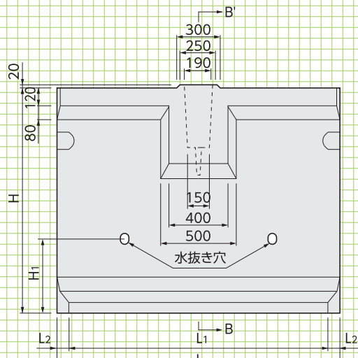
■背面図
