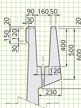
■B-B'断面図
