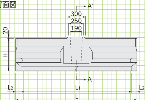
■A-A'断面図
