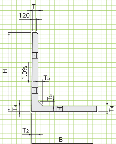
■側面図(90°の場合)
