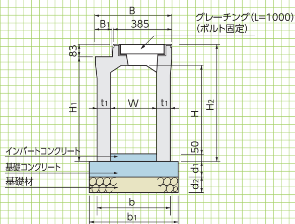
■断面図(W=300,400)
