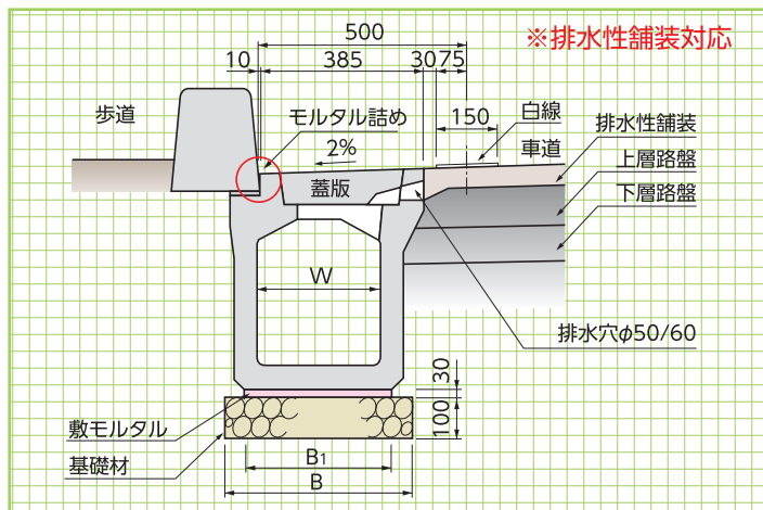
標準敷設図
