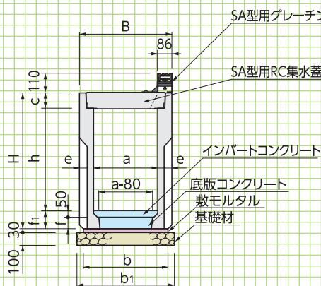
■断面図
