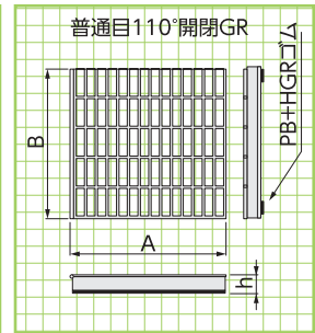
専用グレーチング
