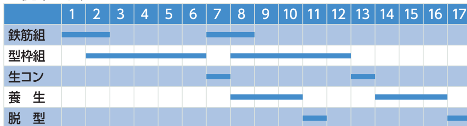
■従来工法
