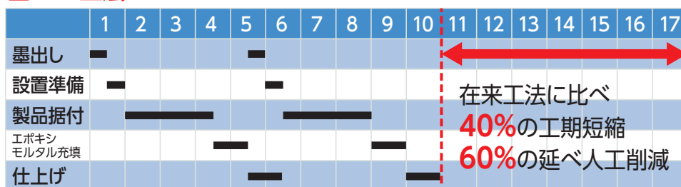
■E&A工法
