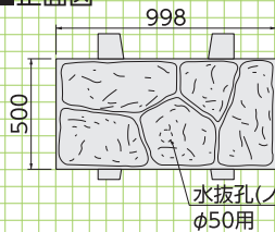
■正面図
