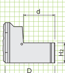
■側面図
