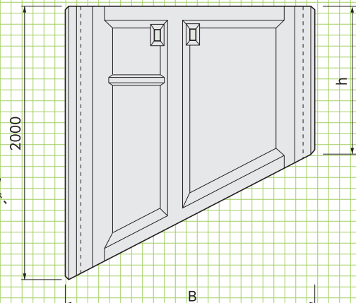
■側面図
