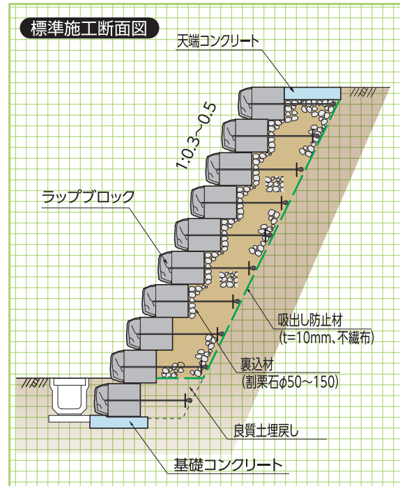
標準断面図
