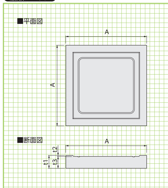
基本形状図
