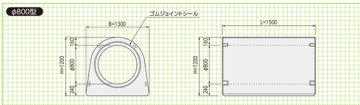
基本形状図 形状・寸法 重量表
