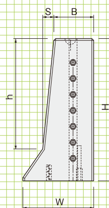
■右側面図
