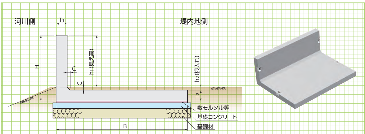
基本形状図
