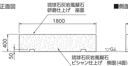
■立面图
