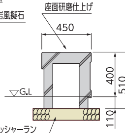
■製品断面図
