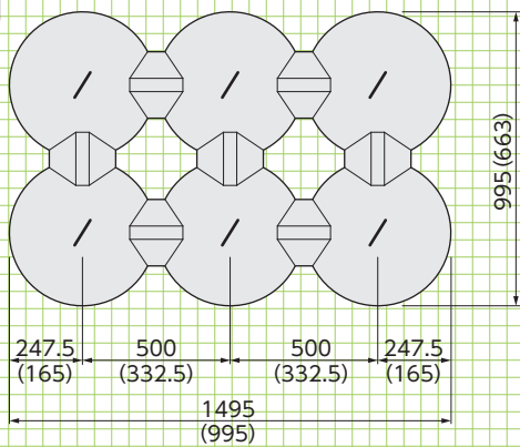
■平面図
