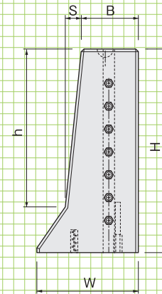
■右側面図
