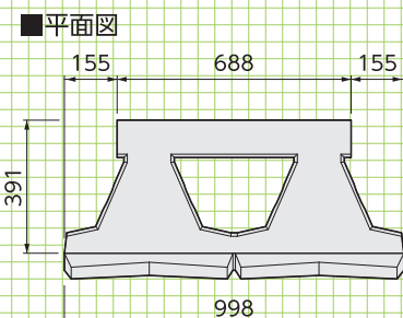
天端ブロック 参考重量:58kg
