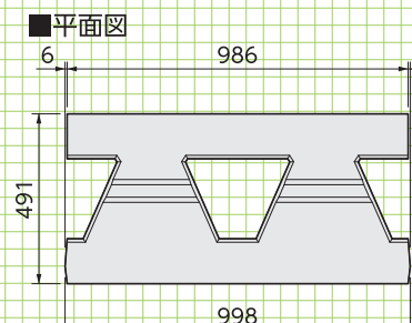
基礎ブロック 参考重量:87kg
