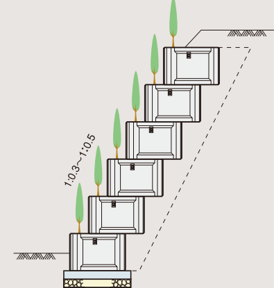
■階段積みもたれ式擁壁
