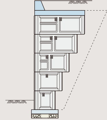
■逆台形式直積み擁壁(RE工法)
