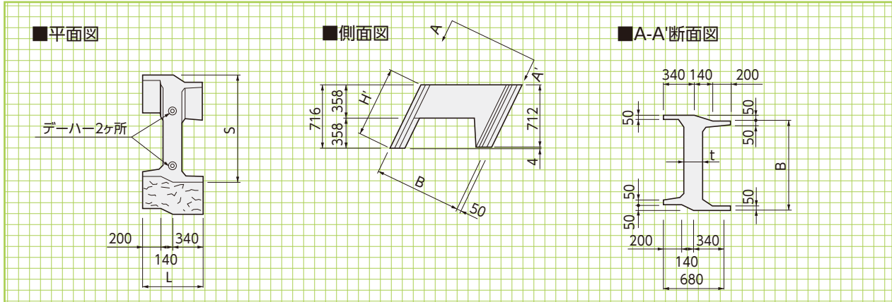
■寸法表(B型)
