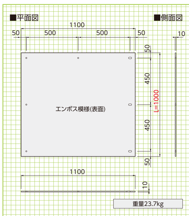
基本形状図
