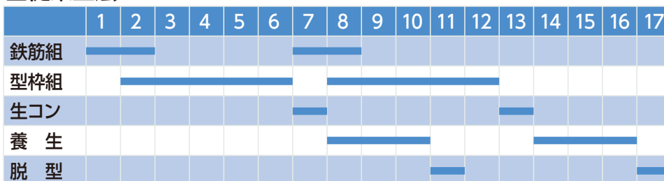
■従来工法
