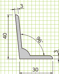
■断面図
