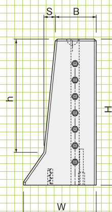
■右側面図
