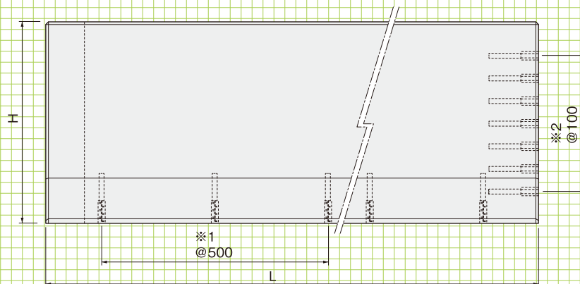
■正面図
