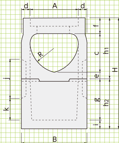
■正面図
