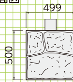
■正面図
