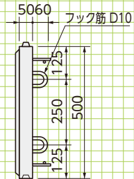
■側面図
