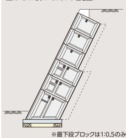
■かさね積みもたれ式擁壁
