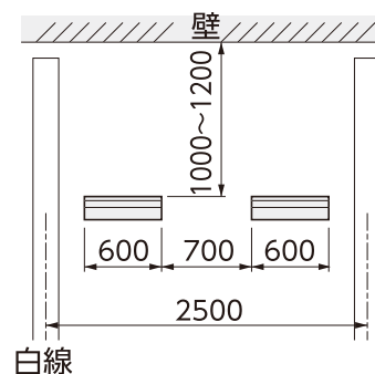
■標準設置図
