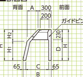
■断面図
