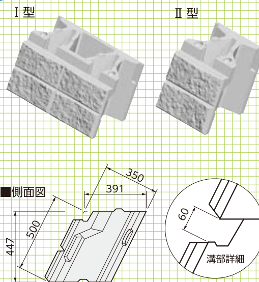
基礎ブロック 参考重量:87kg
