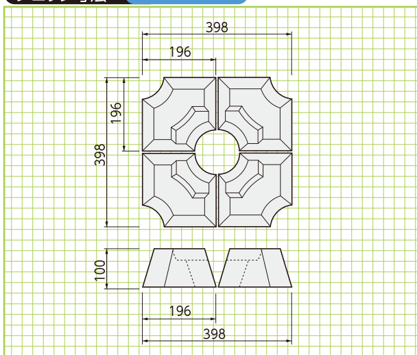
形状・寸法
