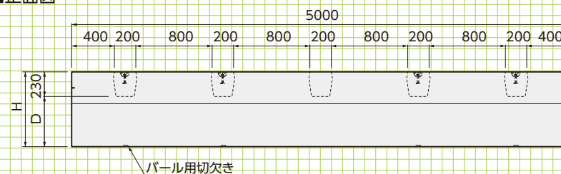
■正面図
