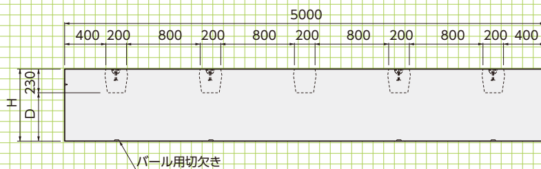
■寸法表(2割勾配用)
