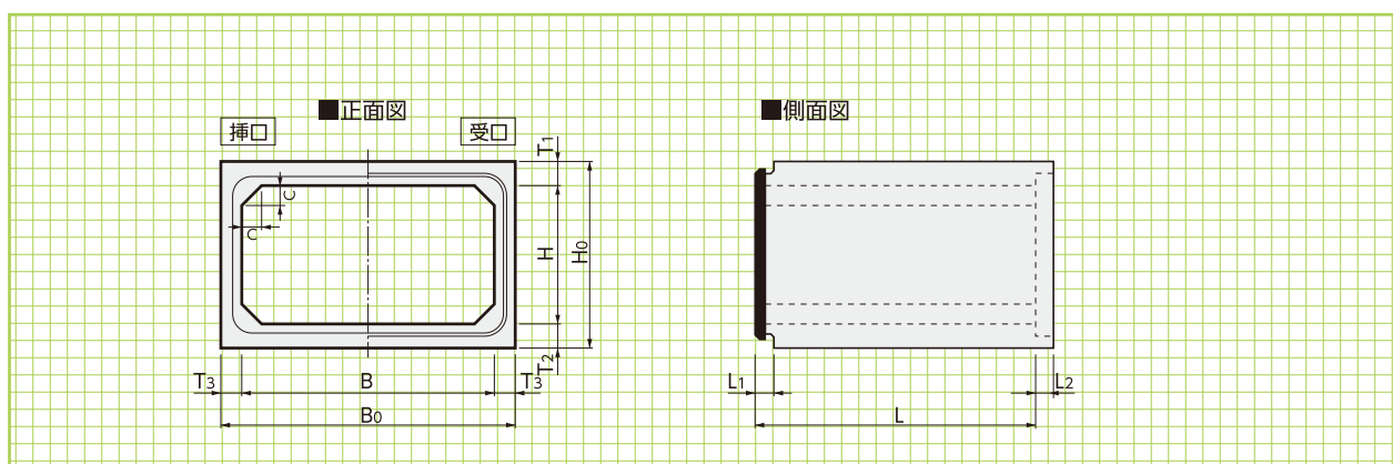
基本形状図
