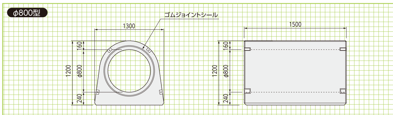
基本形状図
