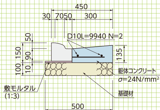
■乗入部断面図
