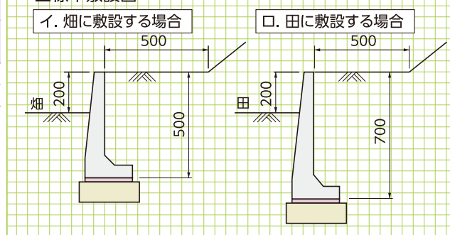
■標準敷設図
