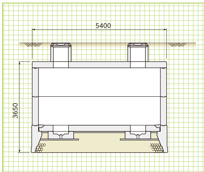
基本形状図
