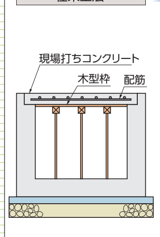
在来工法
