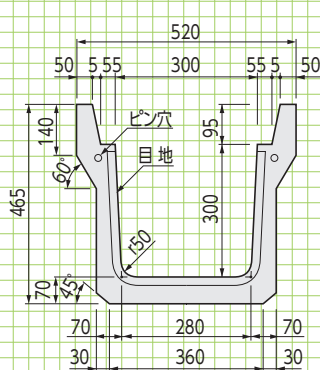
■断面図
