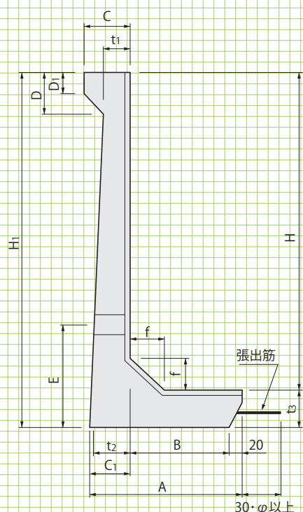
■寸法・重量表
