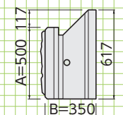
■側面図
