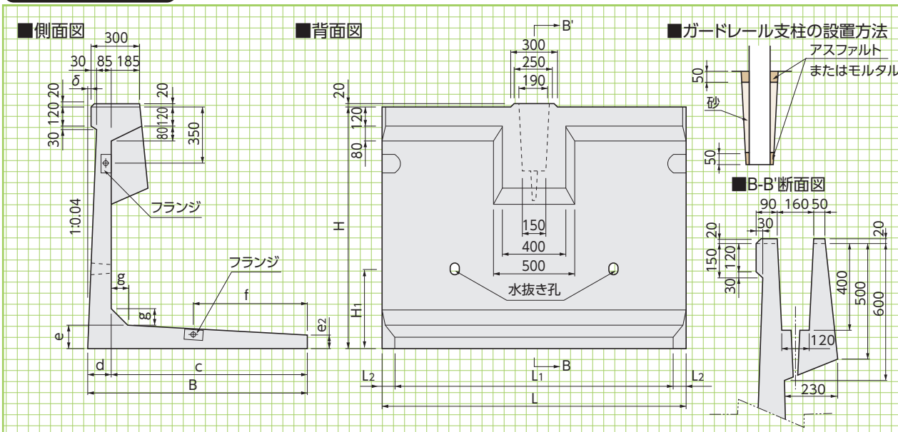
■寸法表 ※( )内数字は外カーブ用です
