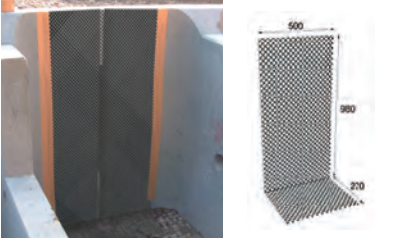
4.L型目地材(ネトロンシート)の設置
