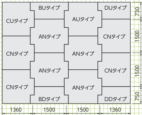
■標準配置設例
