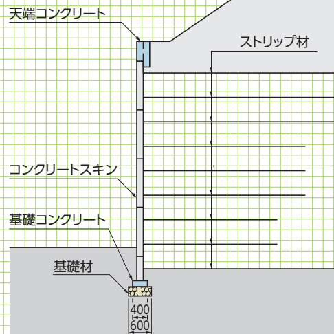
■標準敷設図
