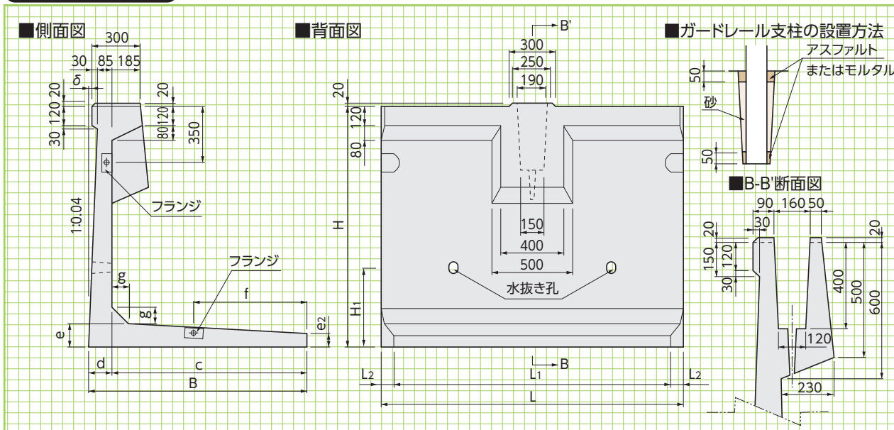
■寸法表 ※(-)内数字は外カーブ用です。 ※(注)800の直線用はございません。 ※L=1500の製品にも対応致します。(端部のみ)
