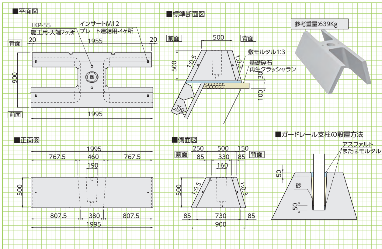
基本形状図
