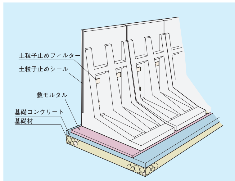
標準敷設図
