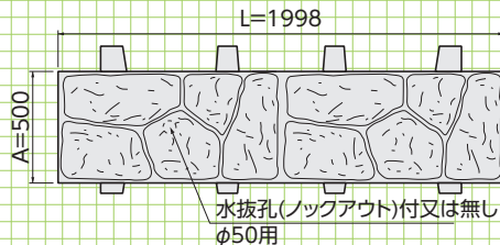
■正面図
