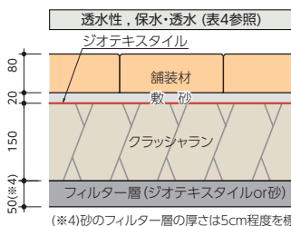
■表 5:歩行者系道路の車両乗入れ部の舗装構造例
