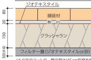
■表 5:歩行者系道路の車両乗入れ部の舗装構造例
