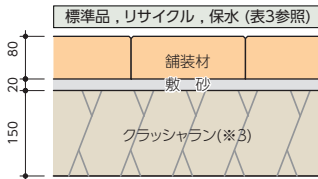
■表 3:乗用車乗入れ部の舗装構造例 【標準品,リサイクル,保水】
