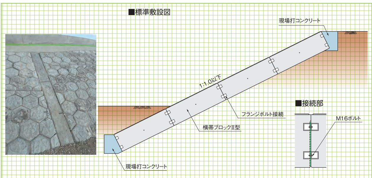
標準敷設図
