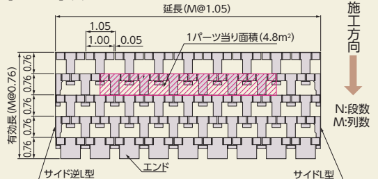
【平面図】(m)
