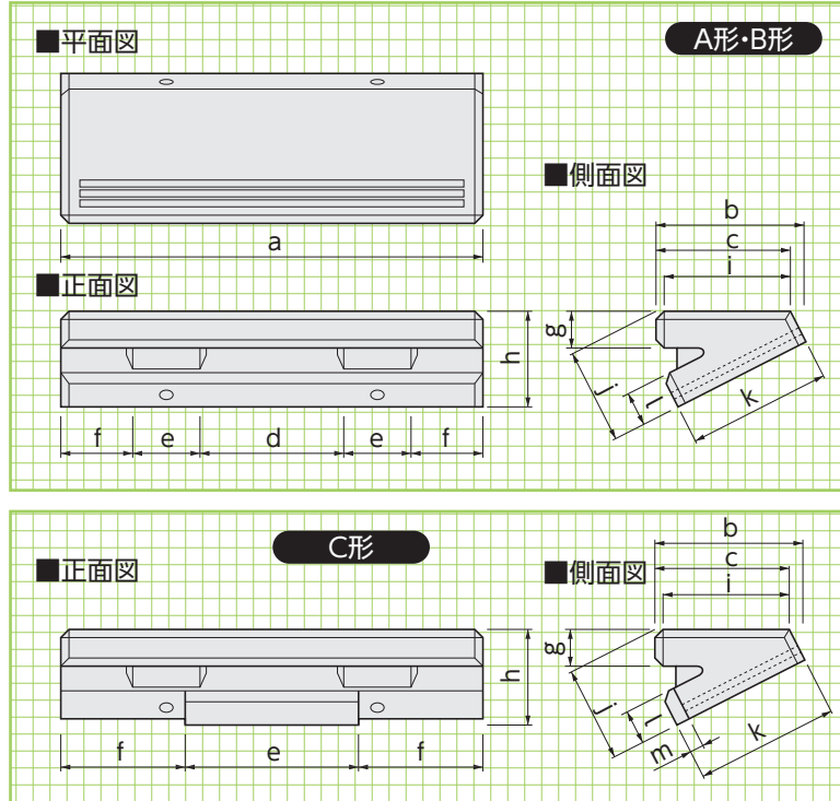
基本形状図
