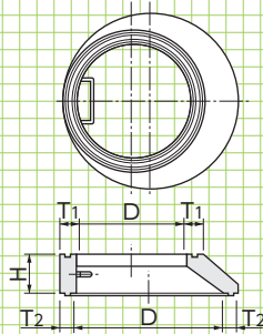
直壁PS
