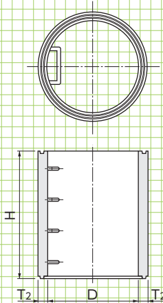
直壁PS
