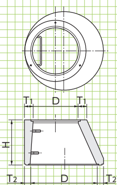
斜壁PT
