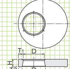
スラブPST
